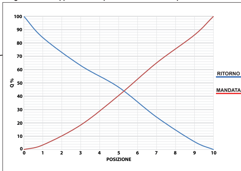
Nel grafico sono rappresentate le portate in funzione della posizione del selettore
